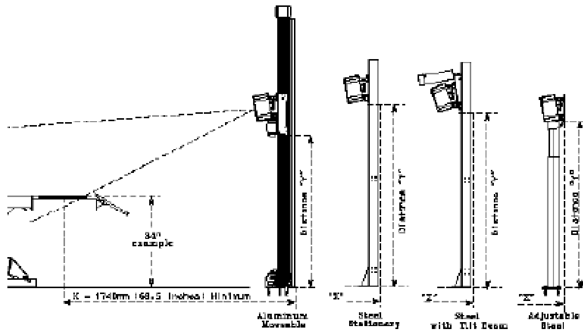
Различные стойки для балки с камерами
